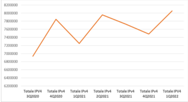
Figura 24 - Situazione Italiana dei dispositivi IPv4 3Q2020, 4Q2020, 1Q2021, 2Q2021, 3Q2021, 4Q2021 e 1Q2022
