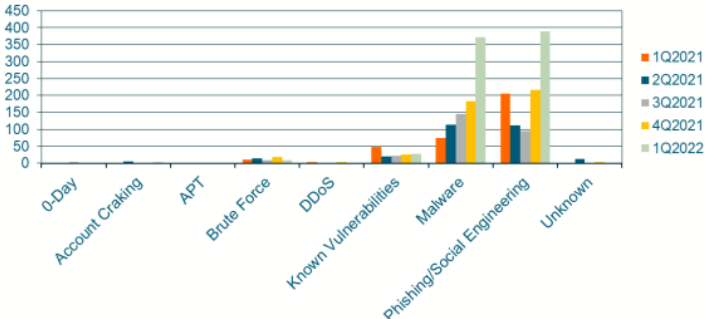
Figura 18 - Tecniche di attacco relative ad attacchi, incidenti e violazioni privacy 1Q2021, 2Q2021, 3Q2021, 4Q2021 e 1Q2022 in Italia
