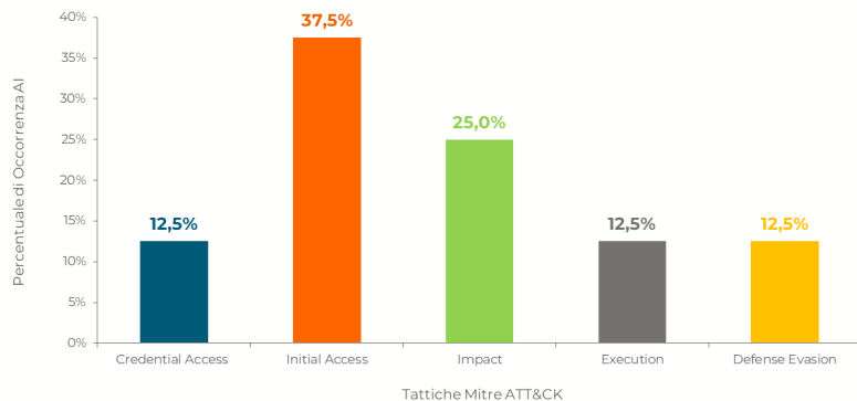
2023 – AI nelle tattiche MITRE ATT&CK®
